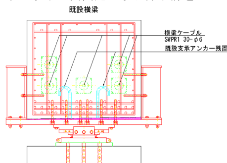
図6 上沓側の既設横梁への取付構造
