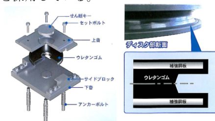
図5 DRB支承
