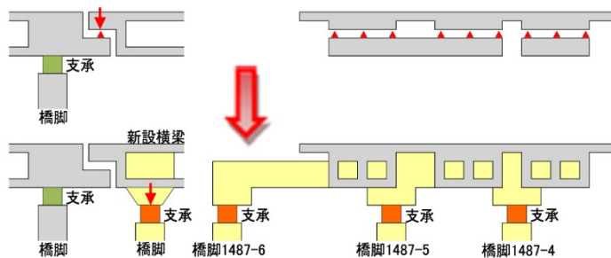
図7 ゲルバー分離部の反力移行イメージ図
