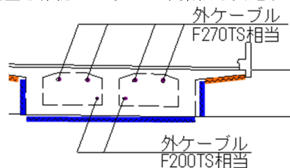
図8 上部工のケーブル配置
