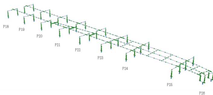
図4 動的解析の立体モデル(1472-1481区間)
