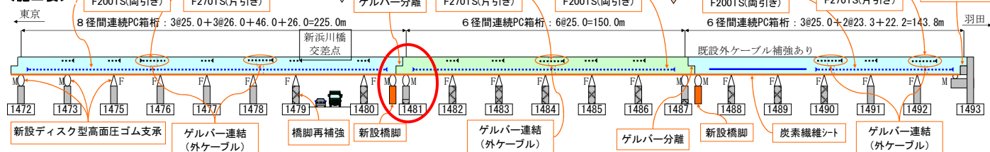
図2 橋梁全体側面図
