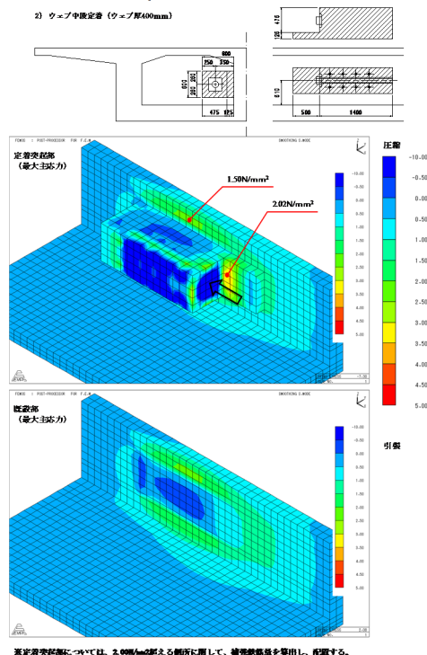
図3 定着突起のFEM解析
