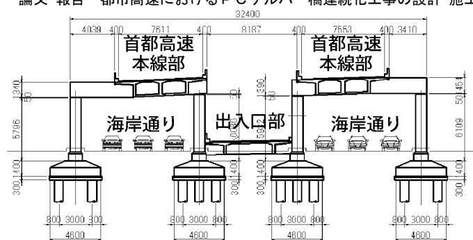
図1 PC箱桁断面図
