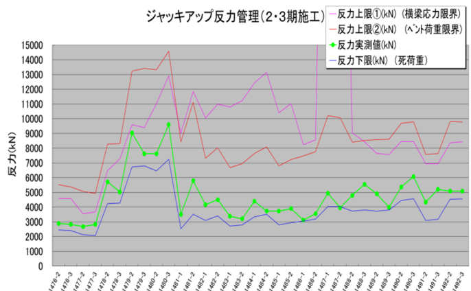
図9 ジャッキアップ反力値（中分側の例）
